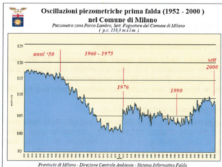
Figura 2.13: Andamento storico del livello piezometrico nella Città di Milano (Prov. Milano, direzione centrale ambiente, servizio acque sotterranee, SIF)
