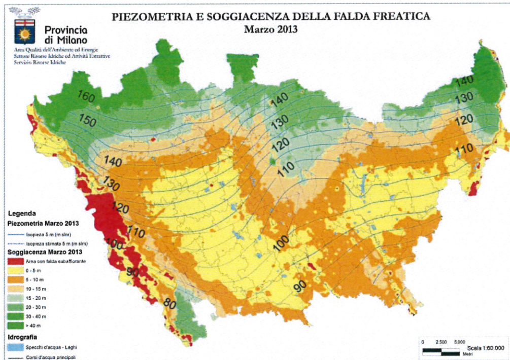
Figura 2.10: Piezometria e soggiacenza della falda freatica registrata nel mese di marzo 2013. Provincia di Milano
