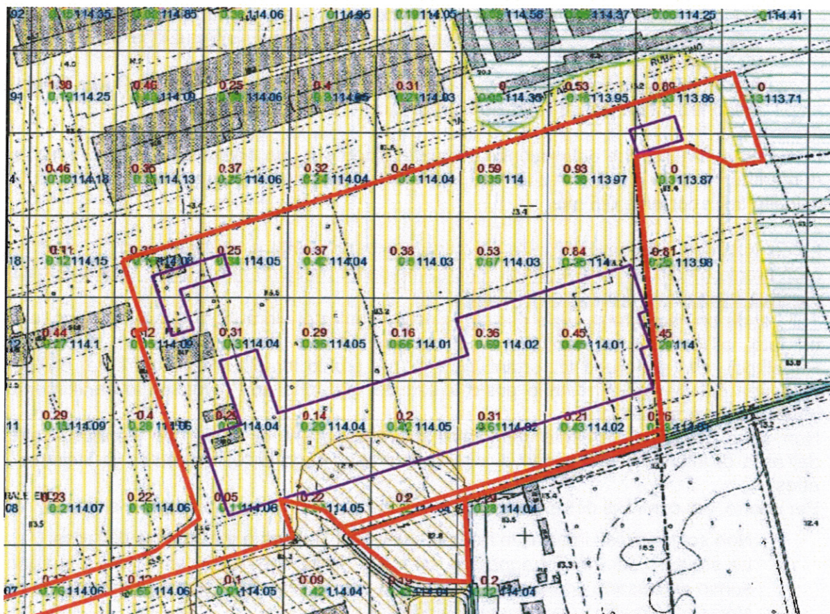
Figura 3.1: dettaglio delle simulazioni idrauliche 2D condotte dal Politecnico di Milano – DIAR per la definizione delle classi di Rischio legate all'esondazione del f. Lambro. Per ogni cella (50x50m) sono definite la quota idrica (blu), il relativo tirante (verde), la velocità della corrente (in rosso).
