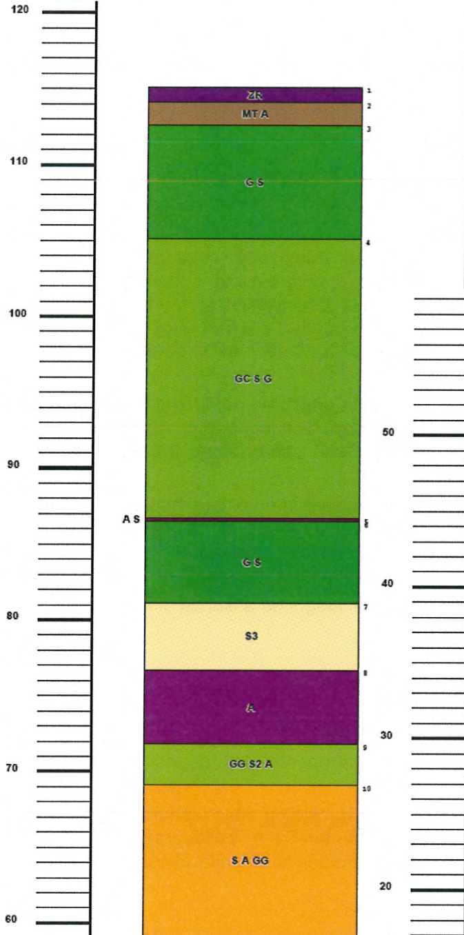
Figura 2.8: Stratigrafia sondaggio geognostico B6C202166096. Servizio Cartografico Regione Lombardia
