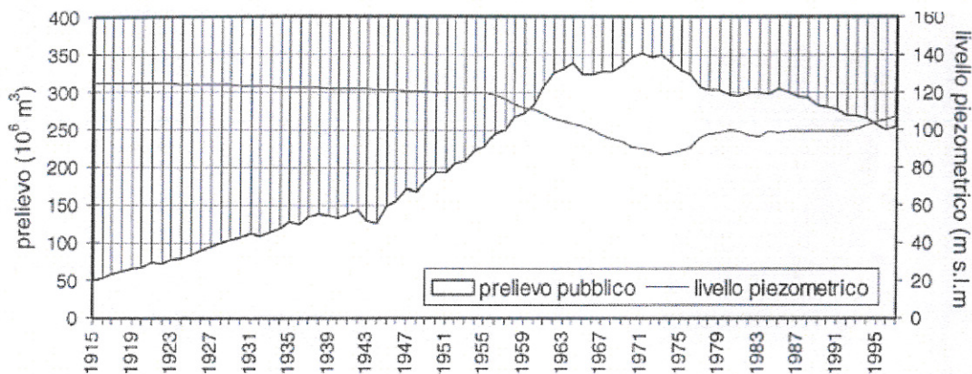
Figura 2.12: Andamento storico del livello piezometrico nella città di Milano (Beretta, 1998)
