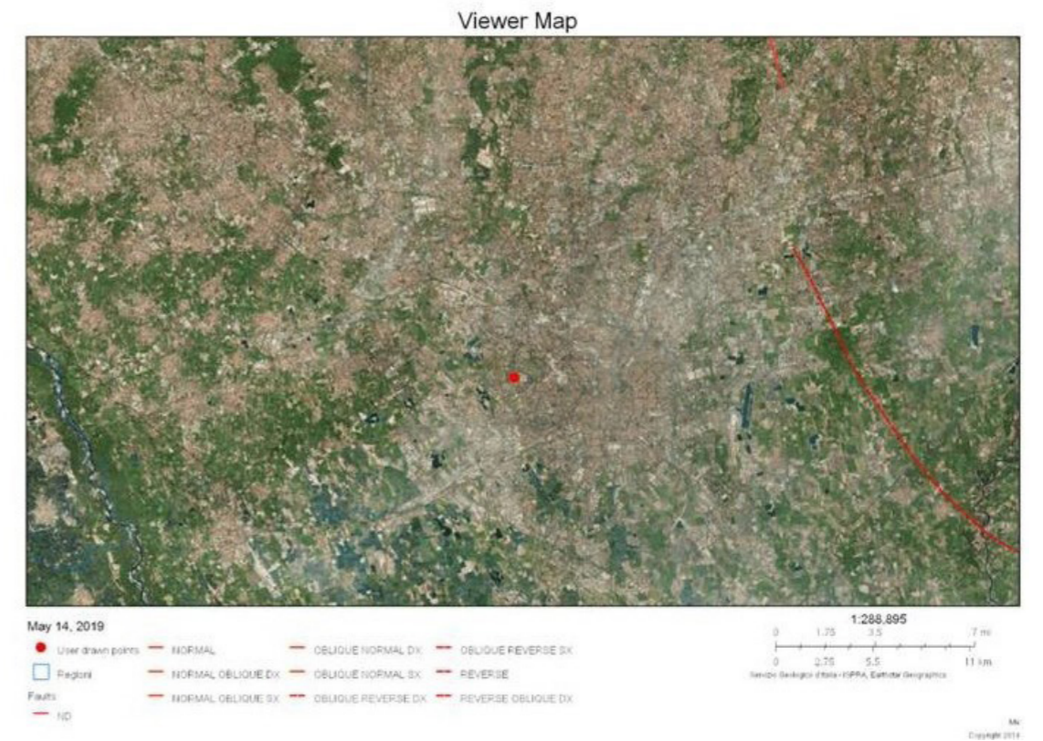
Fig. 05: Faglie capaci (da database ITHACA)
