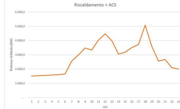
Fig.01: Potenza in KW Riscaldamento e Acqua calda sanitaria
