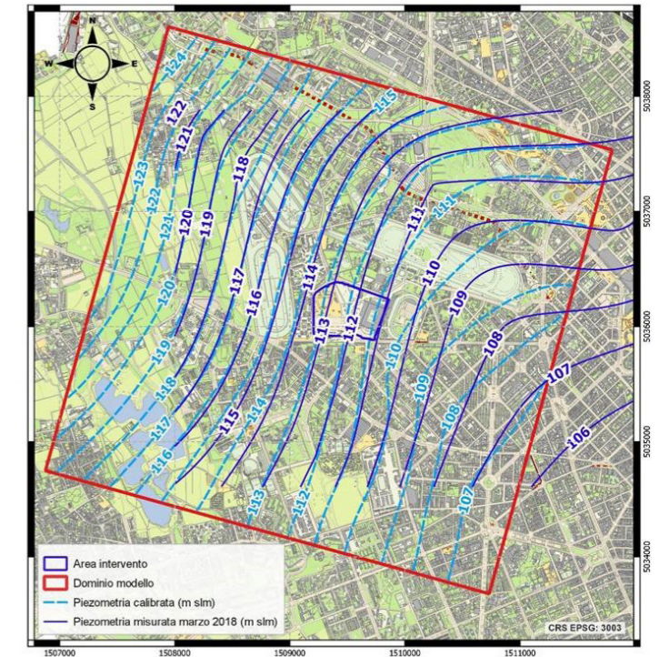
Fig. 11: Confronto piezometria misurata e calibrata
