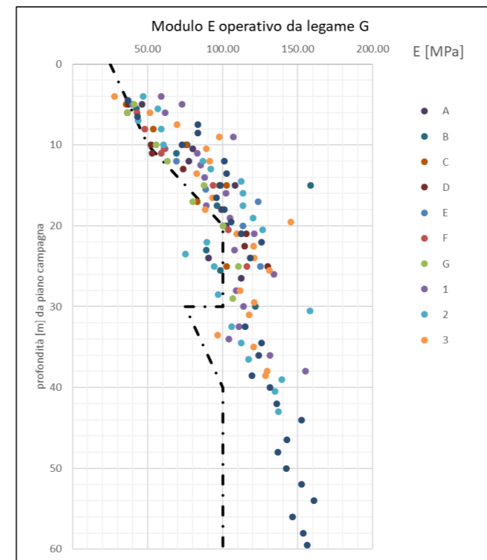
Fig. 10: modulo elastico del terreno - da modulo G
