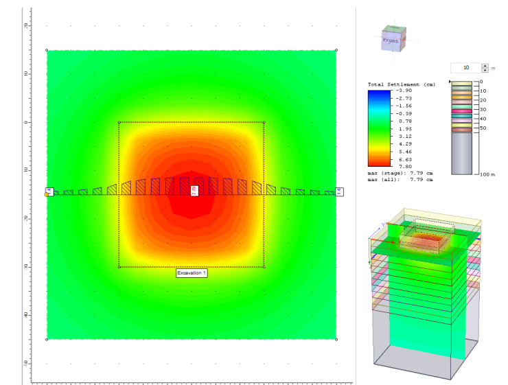
Fig. 20: cedimenti Complesso alberghiero - no strato fine
