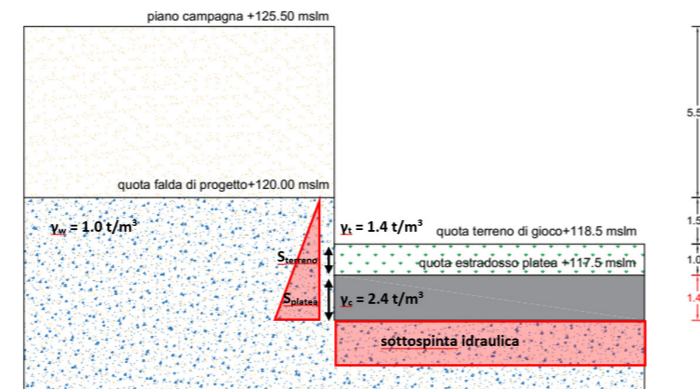
Fig. 22: condizione definitiva del campo di gioco
