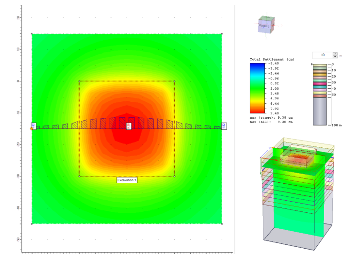
Fig. 21: cedimenti Complesso alberghiero - con strato fine
