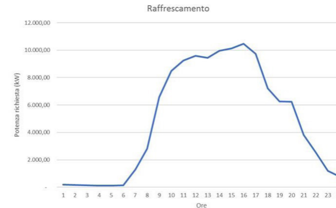
Fig.02: Potenza in KW Raffrescamento
