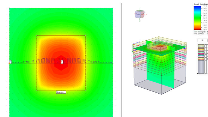
Fig. 18: cedimenti Uffici Est - no strato fine
