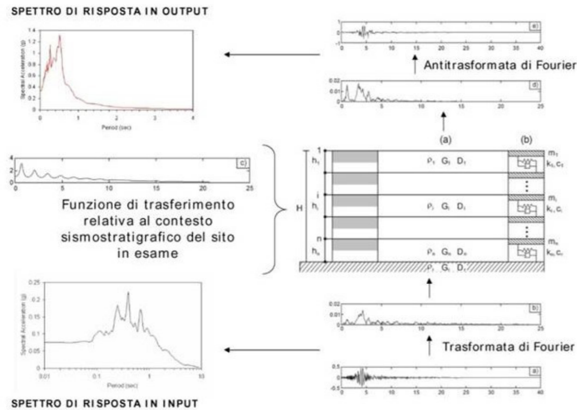
Fig. 08: Diagramma di flusso RSL
