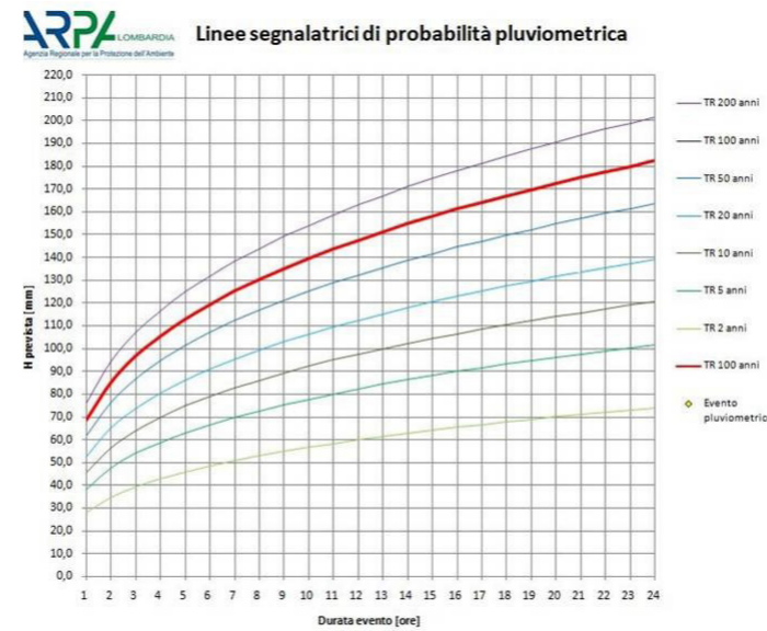
Fig. 07: Curve di possibilità climatica - Tr 100 anni
