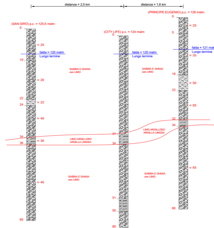
Fig. 12: stratigrafie di riferimento per i siti considerati
