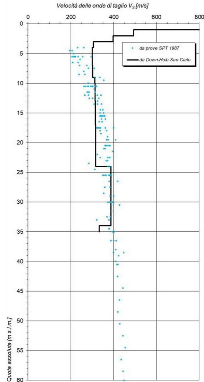
Fig. 09: Stratigrafia V_s
