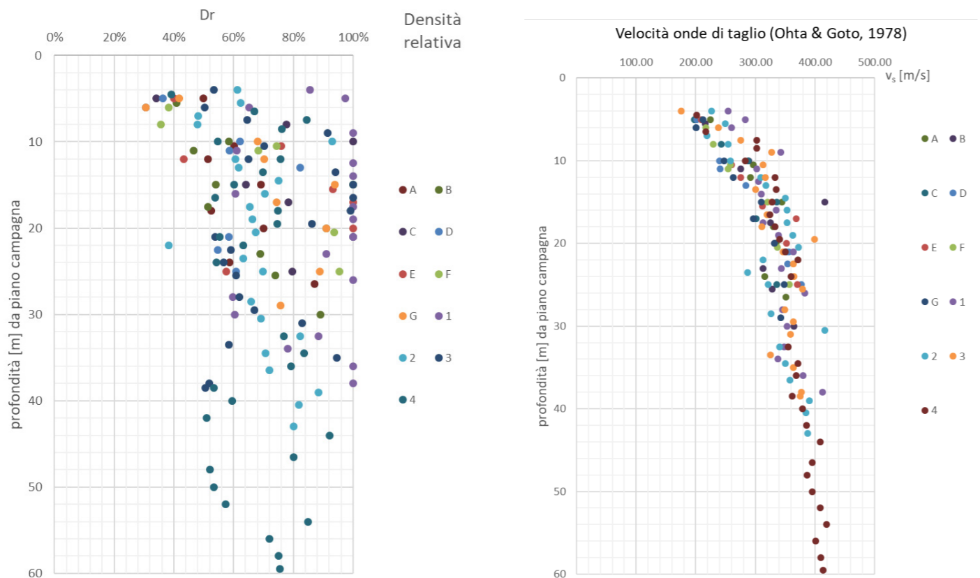
Fig. 06: : densità relativa nei terreni a grana grossa
