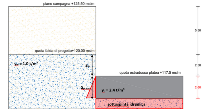
Fig. 24: spessore platea necessaria all'equilibrio con falda di progetto e assenza del terreno di gioco
