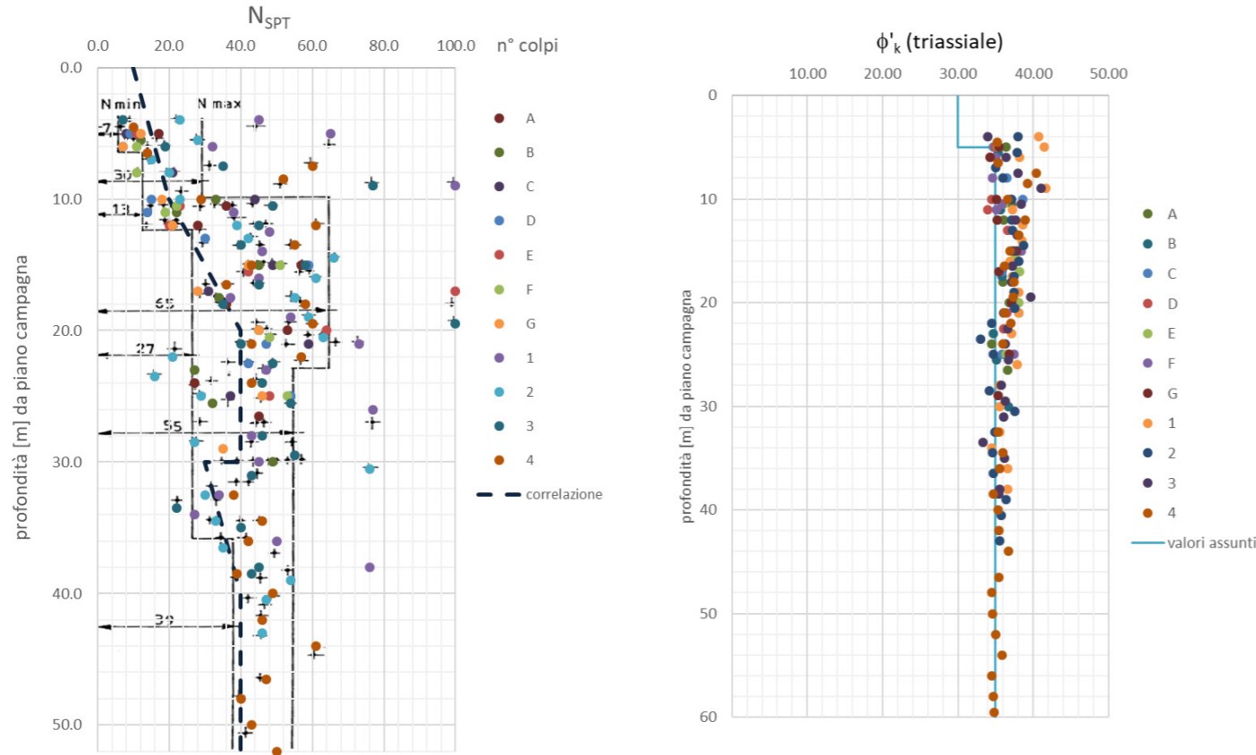
Fig. 05: risultati prove SPT
