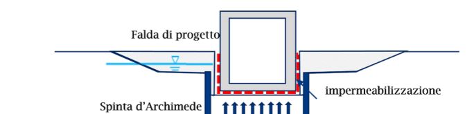
Fig. 16: interazione struttura - falda di progetto
