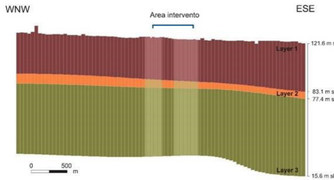
Fig.06: Traccia della sezione idrogeologica (a); sezione idrogeologica (b)
