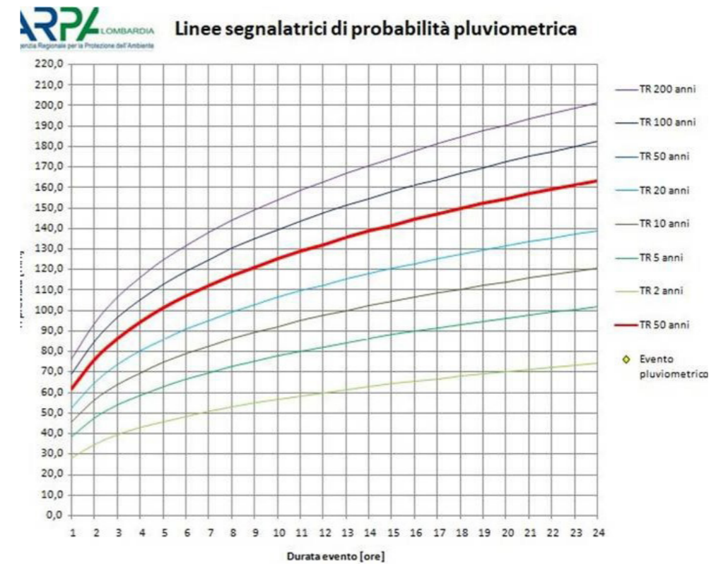
Fig. 03: Curve di possibilità climatica - Tr 50 anni
