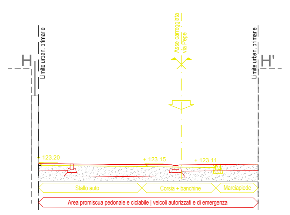
SDF SEZIONE H-H': VIA PEPE - SCALA 1:100
