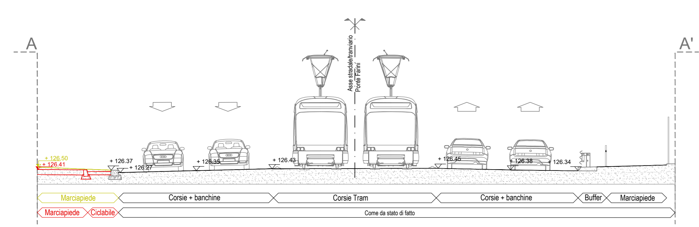
SEZIONE A-A': VIA FARINI - PONTE - SCALA 1:100
