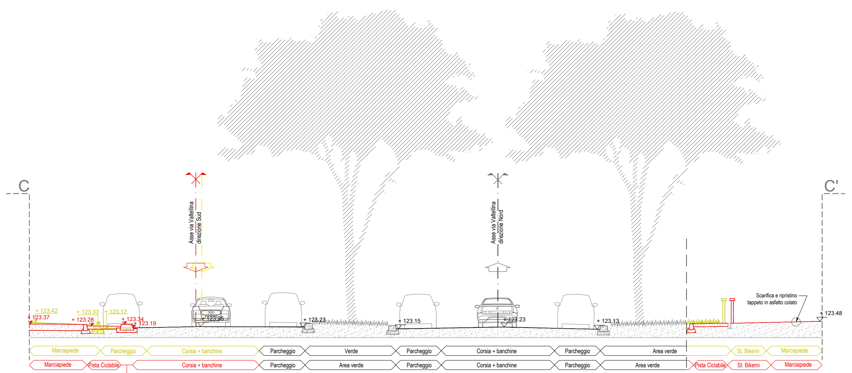
SEZIONE C-C': VIA VALTELLINA - SCALA 1:100
