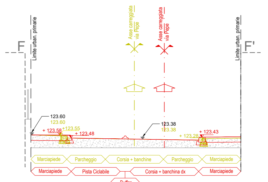
SDF SEZIONE F-F': VIA PEPE - SCALA 1:100
